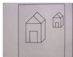
sjena
