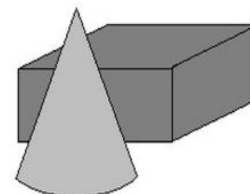
linearna perspektiva
