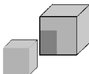
prekrivanje
